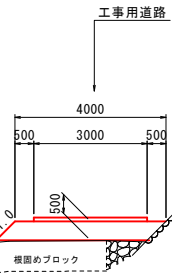
工事用道路断面図 S=1:100
